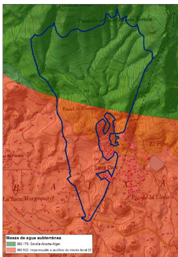
Figura 5.13. Masas de agua subterránea según Plan Hidrológico del Júcar.
