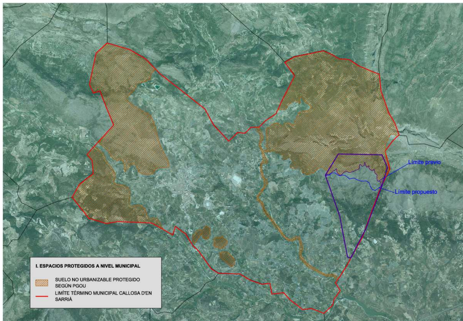
Figura 6.1. Espacios Protegidos a nivel municipal
