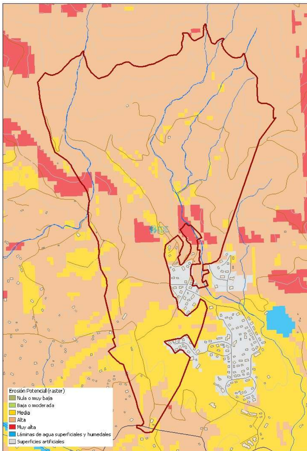
Figura 5.17. Erosión potencial en el ámbito de estudio. Fuente: Catálogo de Servicios Web de Mapas (WMS) de Biodiversidad. MAPAMA.
