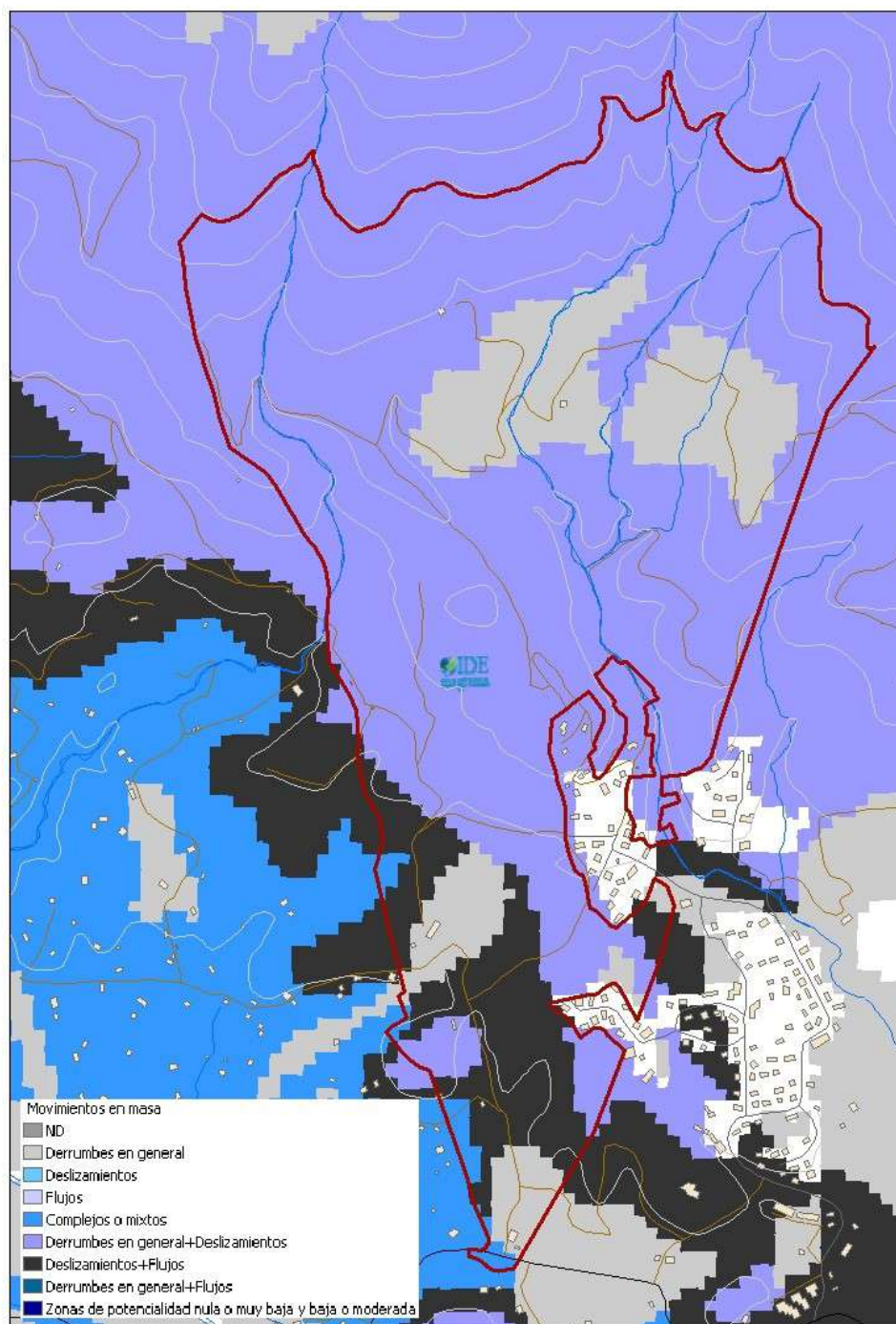
Figura 5.16. Movimientos en masa en el ámbito de estudio. Fuente: Catálogo de Servicios Web de Mapas (WMS) de Biodiversidad. MAPAMA.
