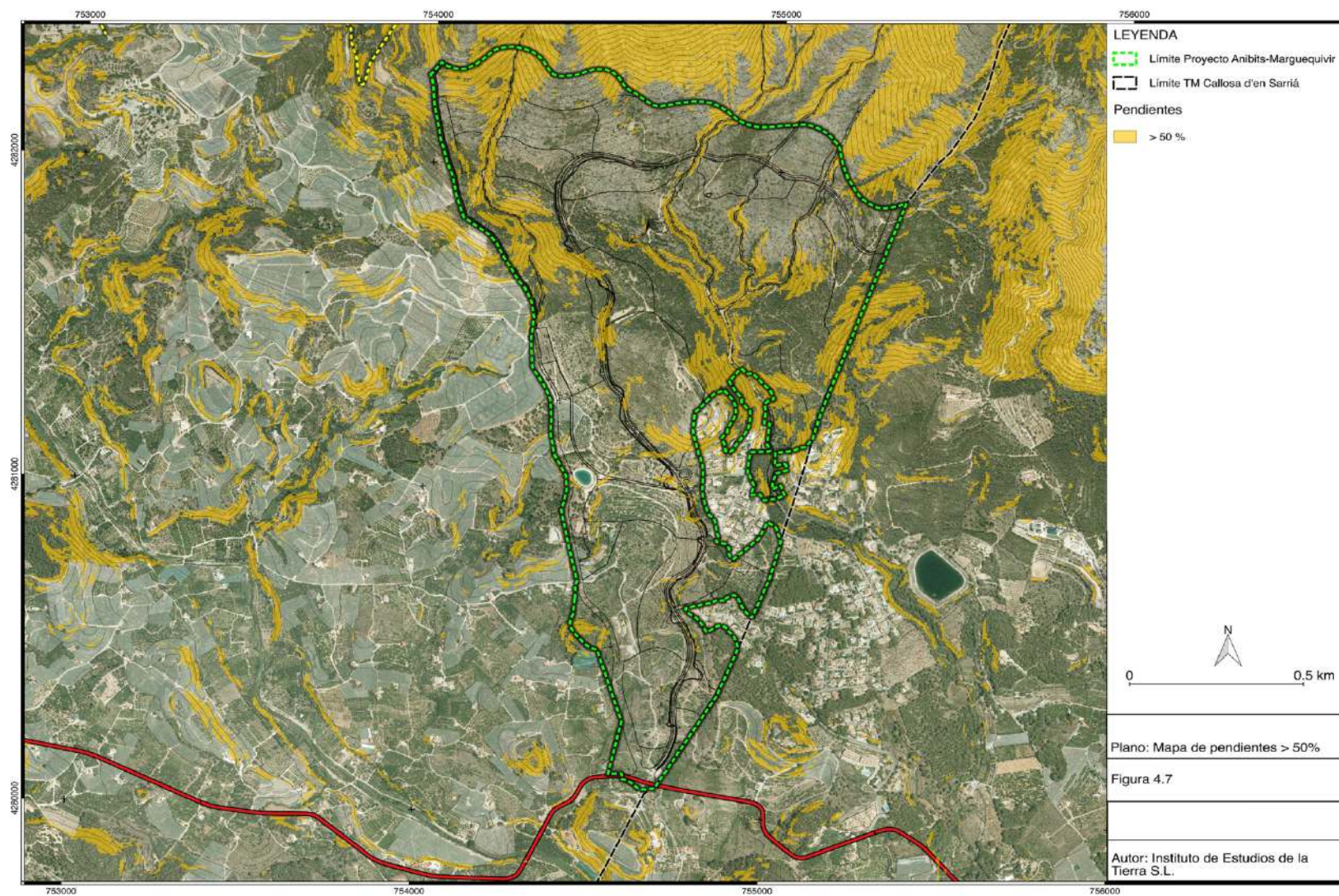
Figura 5.7. Mapa de Pendientes
