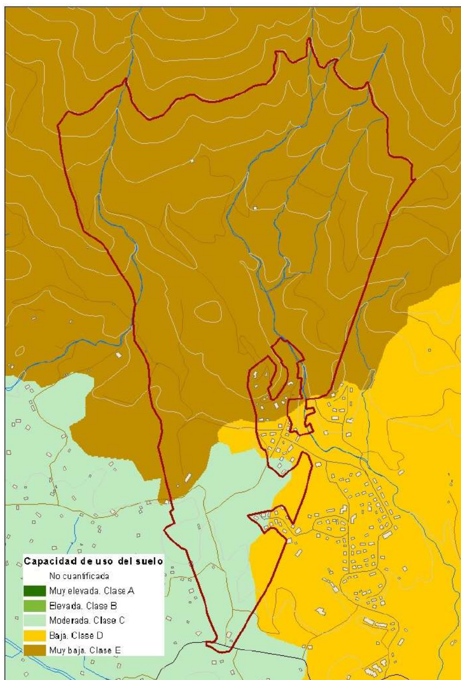
Figura 5.14. Capacidad de uso del suelo en el ámbito de estudio. Fuente: Capacidad de uso del suelo. Generalitat Valenciana.
