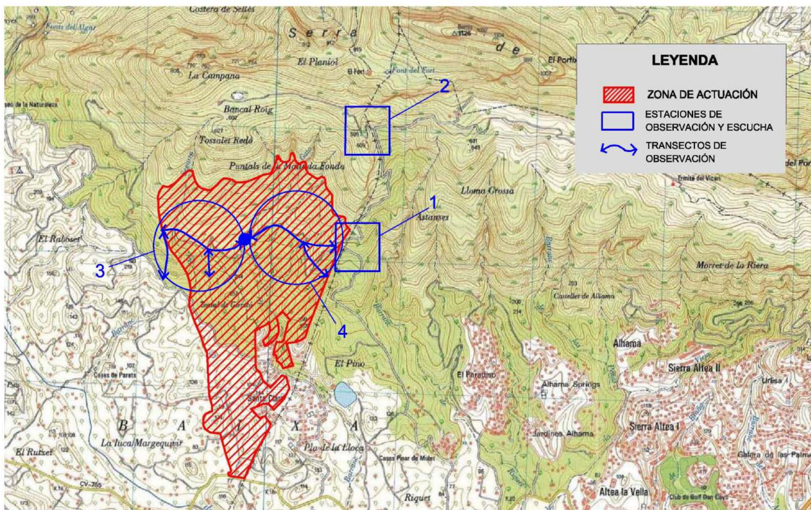
Figura 5.23. Áreas de muestreo de fauna (Muestreo A).
