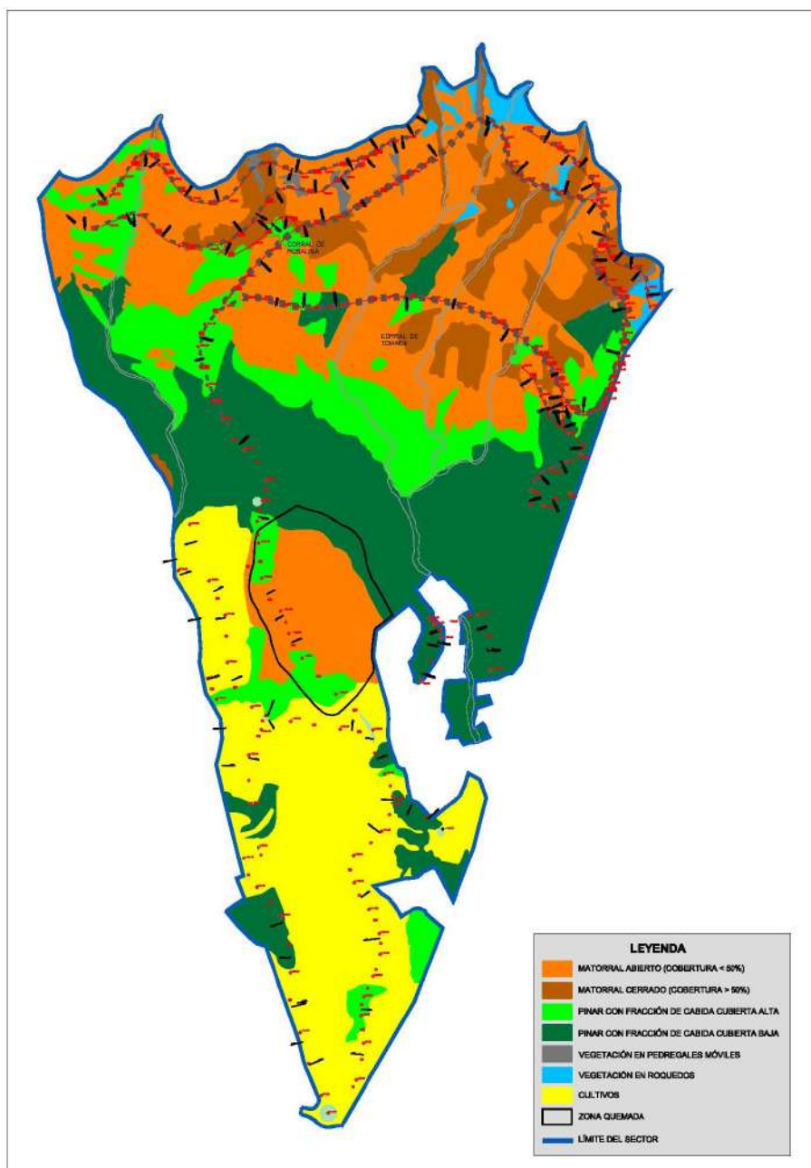
Figura 5.19. Localización de la zona incendiada sobre las unidades de vegetación.
