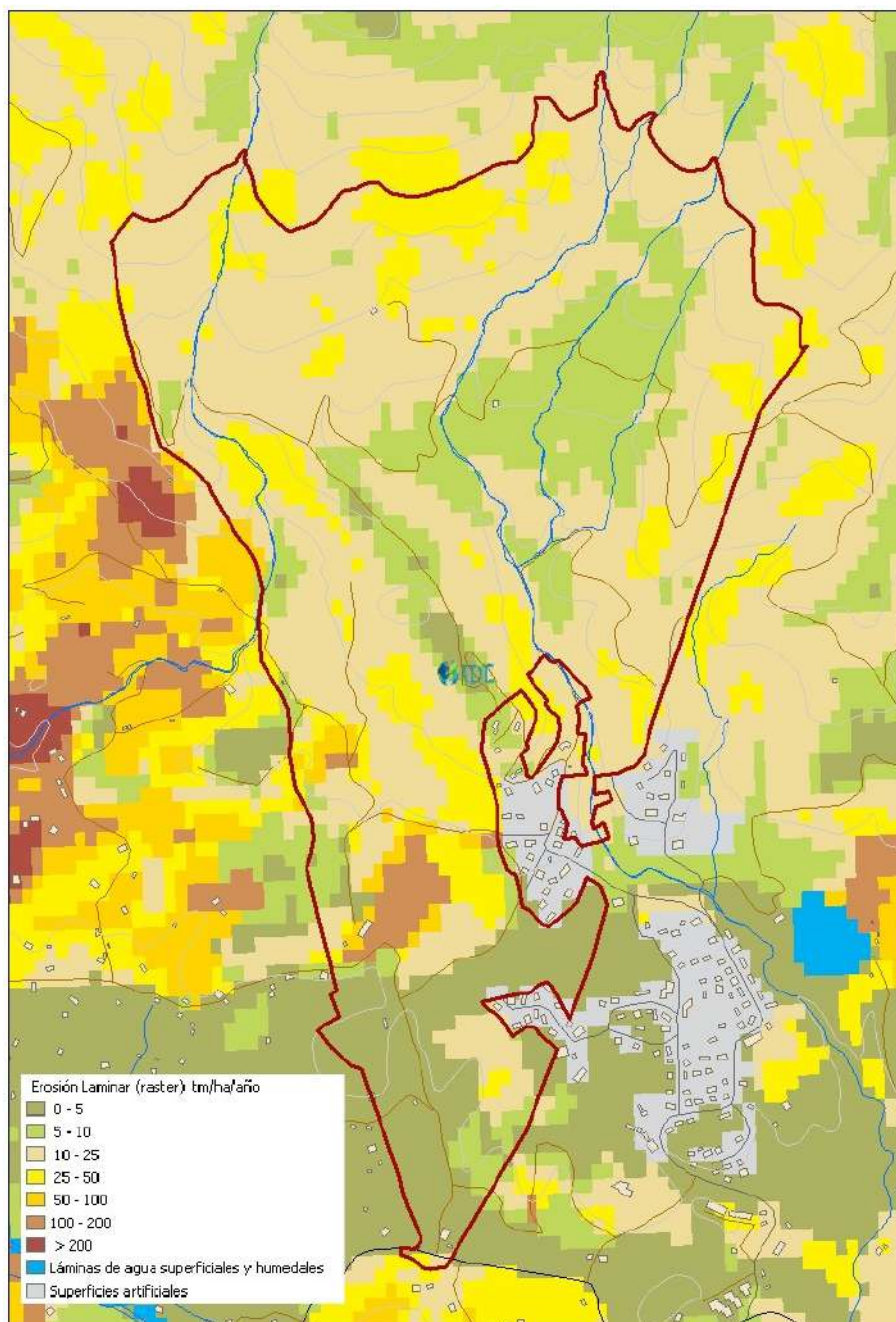
Figura 5.15. Erosión laminar en el ámbito de estudio. Fuente: Catálogo de Servicios Web de Mapas (WMS) de Biodiversidad. MAPAMA
